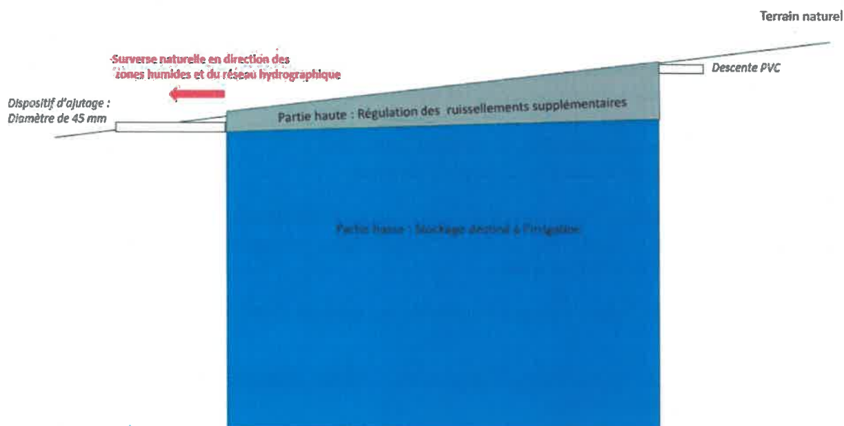
Figure 4 : Schéma de principe du bassin de stockage
